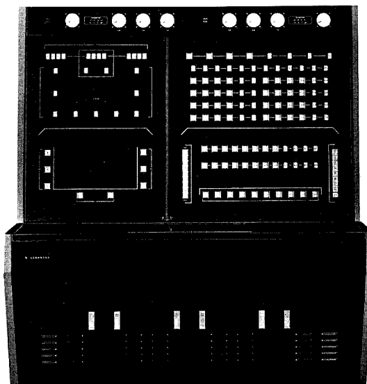
電子クロスバー選択操作盤
