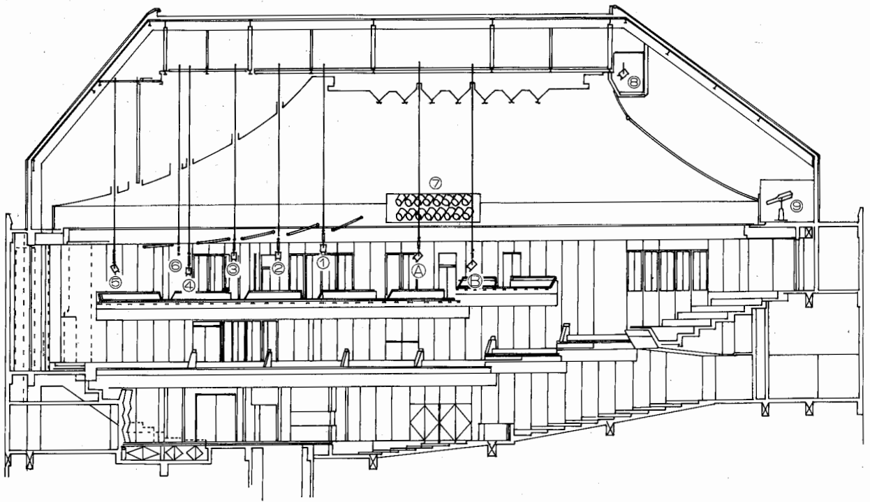
ホール断面図
